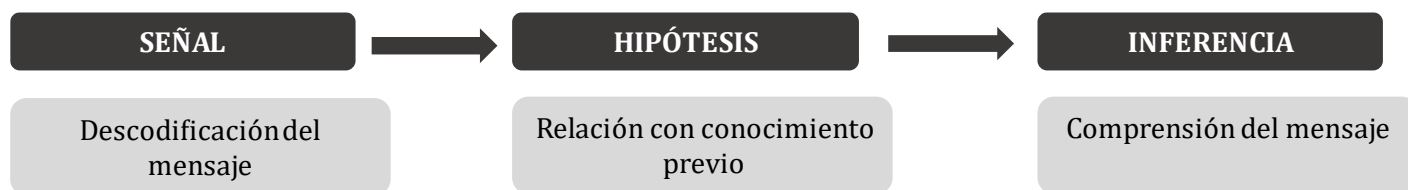
Figura 6. Proceso inferencial
