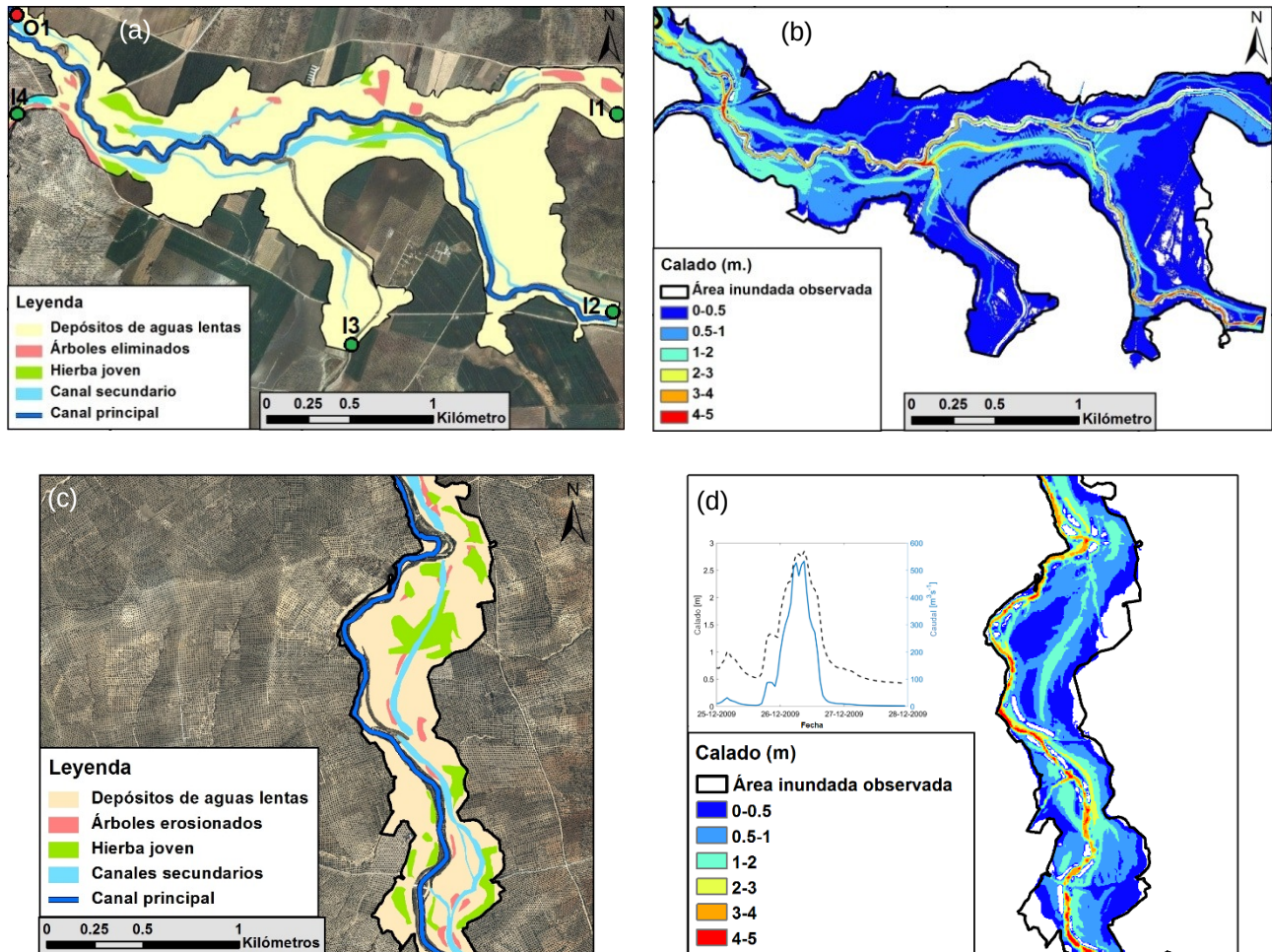
Figura 36. Localización geográfica de las evidencias de paleoinundación remotas localizadas sobre el sector SA13 Arroyo Salado de Arjona (a) y SP13 de Salado de Porcuna (c). (b) y (d) Calado simulado representado sobre el área inundada observada para los mismos sectores (Moral-Erencia et al., 2020).
