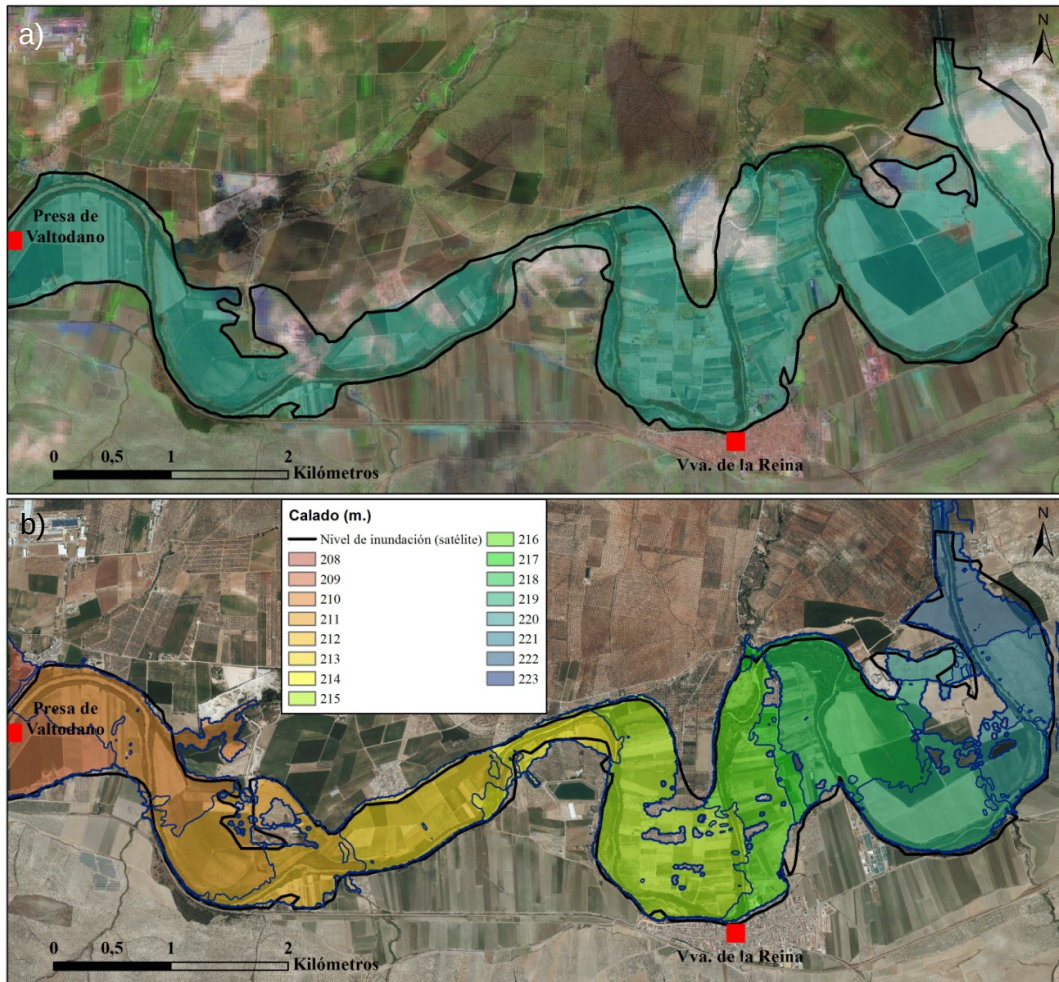
Figura 32. (a) Área inundada observada inferida a partir del satélite Landsat-5 para el día 24 de febrero de 2010 y corregida con fotografías de helicóptero en las zonas donde existe nubosidad. (b) Cota del agua simulada para la misma fecha superpuesta sobre el nivel de inundación observado. Flujo de agua en dirección este-oeste (Bohorquez & del Moral-Erencia, 2017).
