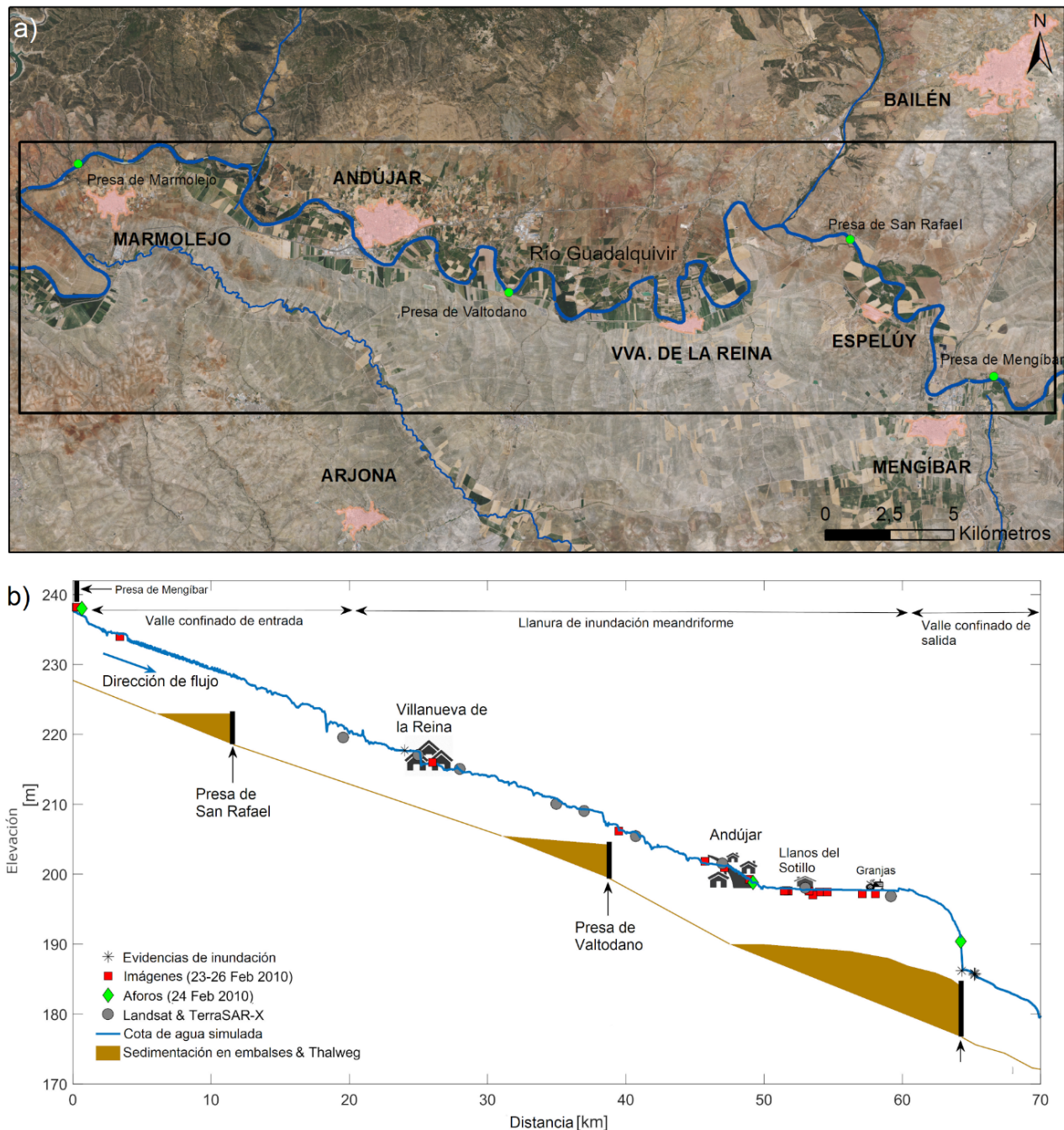
Figura 10. (a) Detalle del sector Mengíbar-Marmolejo del río Guadalquivir. (b) Perfil longitudinal del río Guadalquivir a lo largo del sector Mengíbar-Marmolejo (Bohorquez & del Moral-Erencia, 2017).
