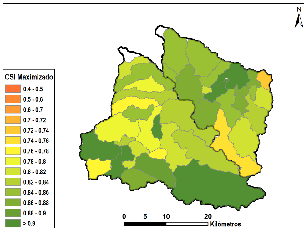
Figura 40. CSI mejorado o maximizado ( CSI_m ) a una escala de subcuenca, obtenido a través de la aplicación recursiva del método desarrollado en esta tesis (Moral-Erencia et al., 2021, enviado).
