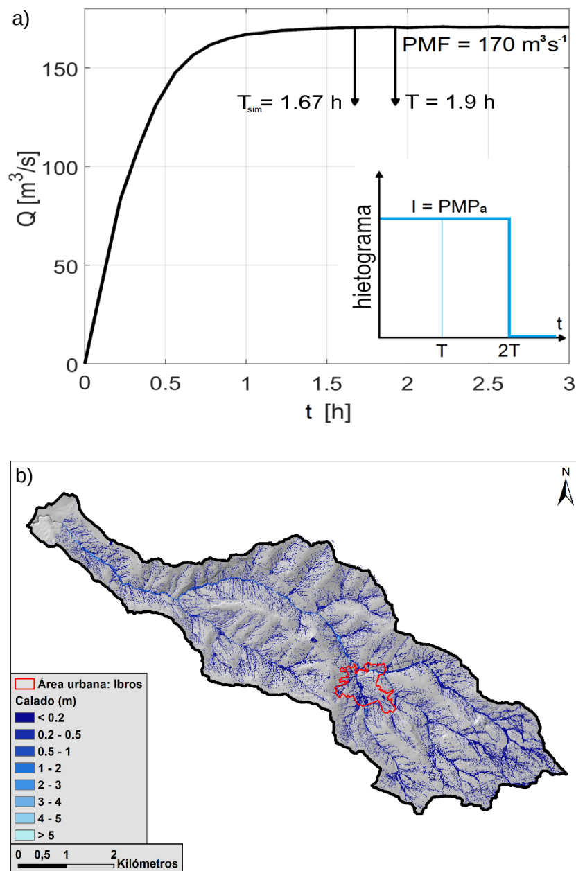
Figura 44. a) Hidrograma derivado del cálculo hidrológico de los procesos de transformación lluvia-escorrentía. Nótese que a t = 1,67 \text{ h} se alcanza el valor inferido de \text{PMF} = 170 \text{ m}^3 \cdot \text{s}^{-1} , próximo al instante 1,9 \text{ h} predicho por el método de la onda cinemática. En la parte inferior derecha se indica el hietograma aplicado en el cálculo hidrológico, dado por \text{PMP}_a durante un período 2T . b) Calado simulado a escala de cuenca (m). Es de destacar las intensas escorrentías producidas en la inundación relámpago que son canalizadas a lo largo de la cuenca por la red de drenaje, afectando directamente a las áreas urbanas (perímetro rojo) (Moral-Erencia et al., 2020).
