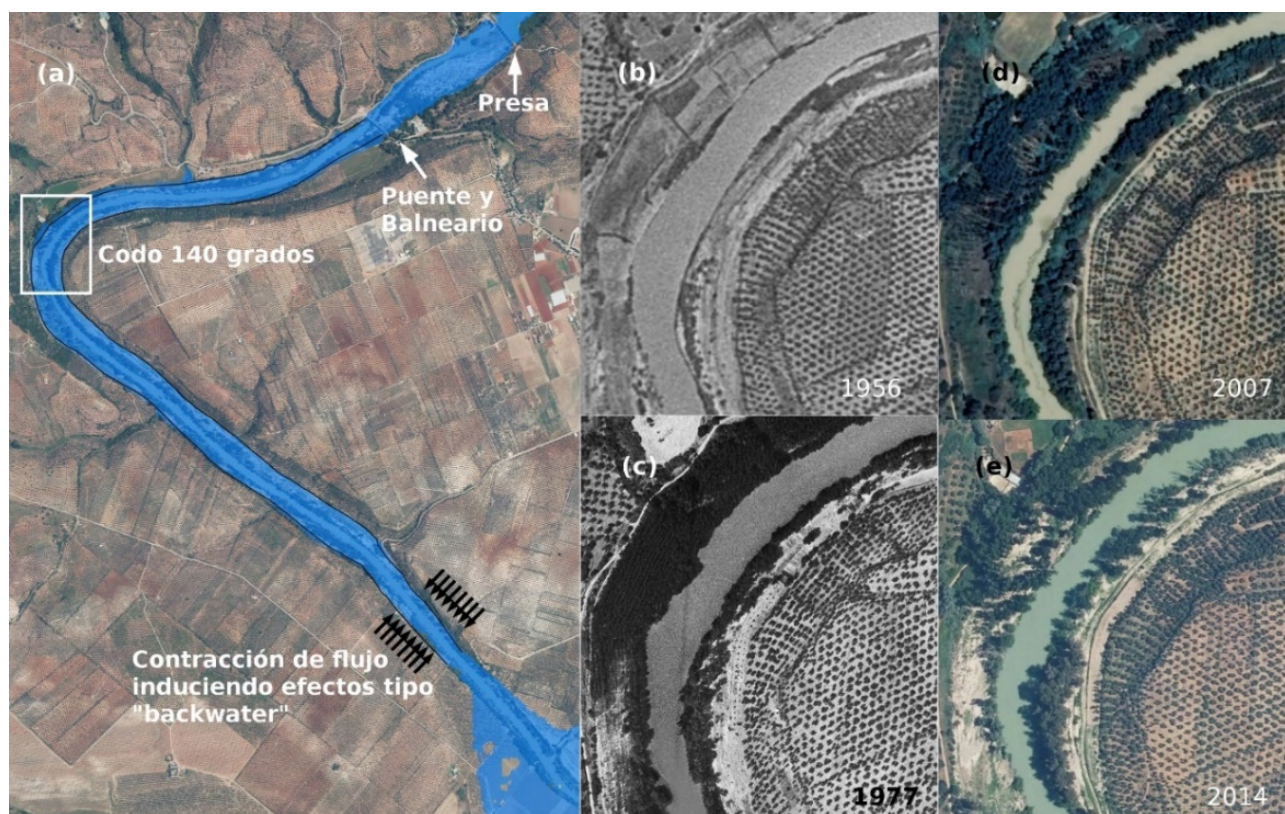
Figura 31. (a) Relleno en color azul representando el área inundada simulada para una descarga de 1.400 \text{ m}^3 \cdot \text{s}^{-1} con un coeficiente de rugosidad de 0,05 \text{ s} \cdot \text{m}^{-1/3} . (b)–(e) Secuencia de ortofotografías mostrando el estado anterior y posterior a la regulación fluvial (1956 - 2014).
