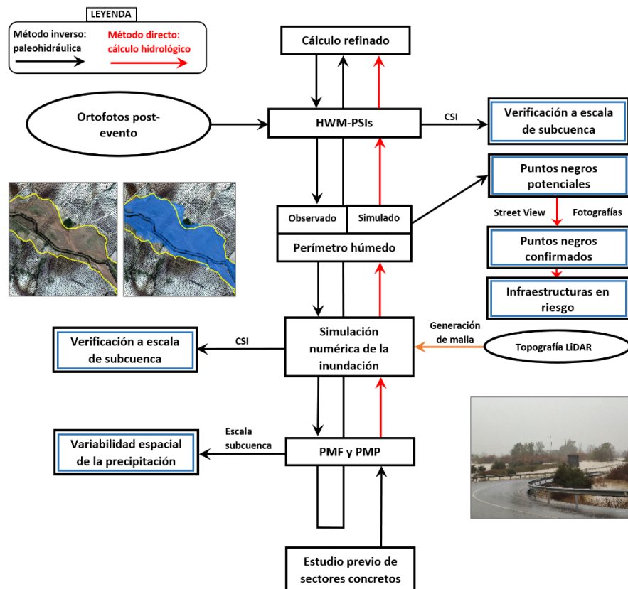
Figura 34. Diagrama de flujo resumiendo la aplicación del método inverso (flechas negras) y directo (flechas rojas) a lo largo del presente apartado. Un paso común en ambos procedimientos se indica con una flecha naranja (Moral-Erencia et al., 2021, enviado).
