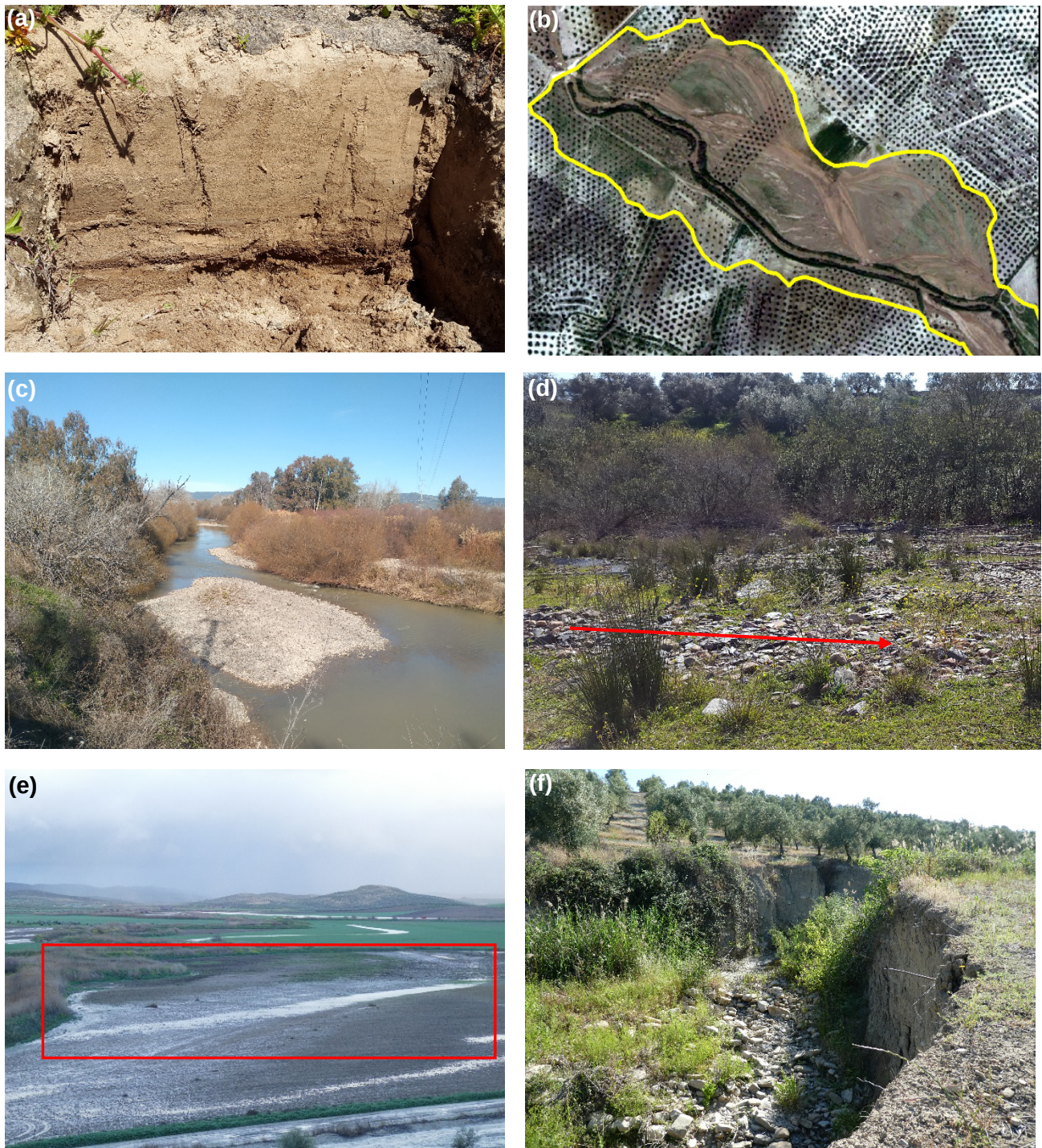
Figura 17. (a) Corte trasversal de un depósito de aguas lentas en el que se aprecia la secuencia cronoestratigrafía de una inundación. (b) Depósitos de aguas lentas sobre la llanura de inundación del arroyo Salado de Porcuna tras la inundación de lluvia corta de diciembre de 2009, perfectamente observables desde una ortofotografía del satélite WorldView-1. (c) Barra sedimentaria de granulometría gravosa presente sobre el río Guadalquivir. (d) Imbricación de clastos en el sentido del flujo en un paraje aledaño al río Guadalquivir. (e) Tallado de canales secundarios (recuadro rojo) en la llanura de inundación del arroyo Salado de Arjona. (f) Desarrollo de importantes procesos de erosión lateral en el arroyo de Ibros.
