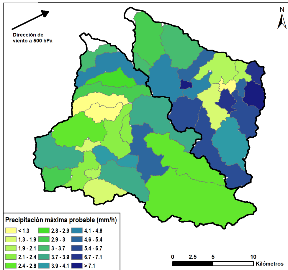
Figura 41. Precipitación máxima probable ( \text{mm} \cdot \text{h}^{-1} ) en las cuencas SP y SA para el evento de inundación de lluvia corta comprendido entre 26 y 27 de diciembre de 2009. Podemos observar una distribución heterogénea de la tasa de precipitación. En la parte superior izquierda se indica la dirección del viento a 500 hPa ( \sim 5500 m) del reanálisis NOAA GDAS (Kalnay et al., 1996) en el momento pico de precipitación (Moral-Erencia et al., 2021, enviado).
