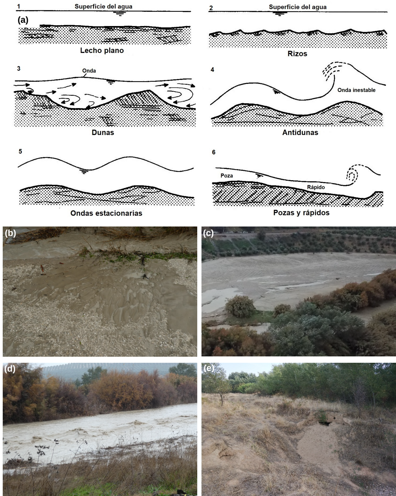
Figura 18. (a) Diagrama esquemático de las principales forma de lecho fluvial (adaptado de Simons & Richardson, 1966). (b) Rizos formados sobre una infraestructura viaria próxima al Arroyo Salado de Arjona. (c) Campo de dunas desarrollado tras una inundación de lluvia corta. (d) Antidunas desarrolladas en el Arroyo Salado de Porcuna durante la inundación de lluvia corta de diciembre de 2019. (e) Poza erosionada sobre la llanura de inundación del río Guadalquivir durante las inundaciones de lluvia larga de febrero de 2010.
