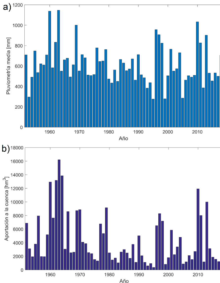
Figura 6. (a) Precipitación media anual (mm) y (b) aportaciones propias acumuladas (hm 3 ) en la cuenca de drenaje del río Guadalquivir durante el período 1951 – 2018.
