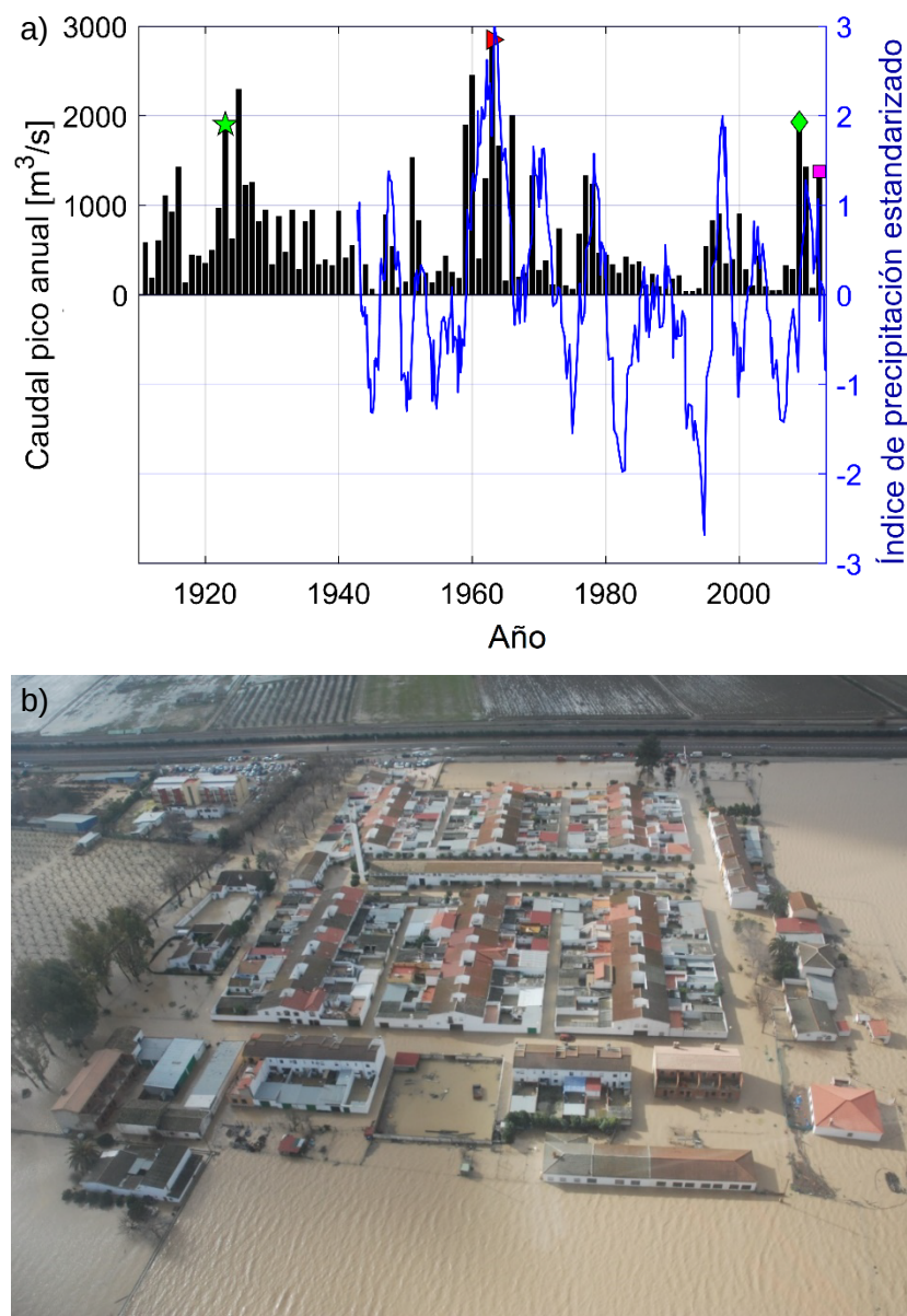
Figura 11. (a) Caudal pico anual registrado en el aforo de Marmolejo (años 1912 – 2015) (barras de color negro) e índice de precipitación estandarizado (SPI) de 36 meses (1942 – 2015) (Bohorquez & del Moral-Erencia, 2017). (b) Imagen de helicóptero de la inundación del río Guadalquivir producida en febrero de 2010 sobre la pedanía de Llanos del Sotillo (Andújar).
