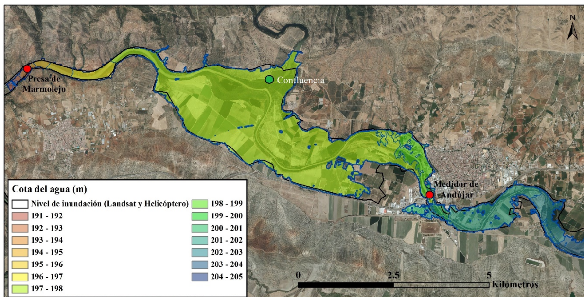
Figura 33. Simulación numérica de la inundación (contornos en color) y área inundada obtenida a partir de los satélites Landsat/TerraSAR-X e imágenes de helicóptero para el día 24 de febrero de 2010. Se indican los aforos de Andújar y la presa de Marmolejo con un punto rojo. La confluencia entre el río Jándula y el Guadalquivir se destaca con un punto verde (Bohorquez & del Moral-Erencia, 2017).
