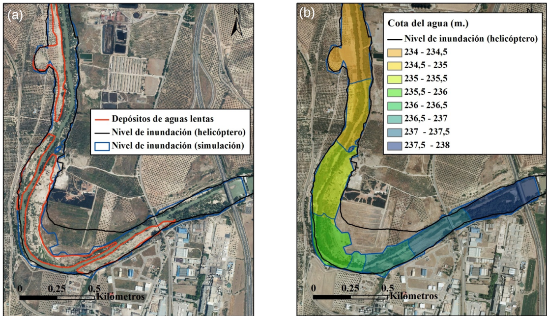
Figura 27. (a) Área observada y simulada de la inundación, junto a los depósitos de aguas lentas (SWD) identificados. (b) Cota simulada de la superficie de agua. El flujo del agua discurre de este a oeste (Bohorquez & del Moral-Erencia, 2017).
