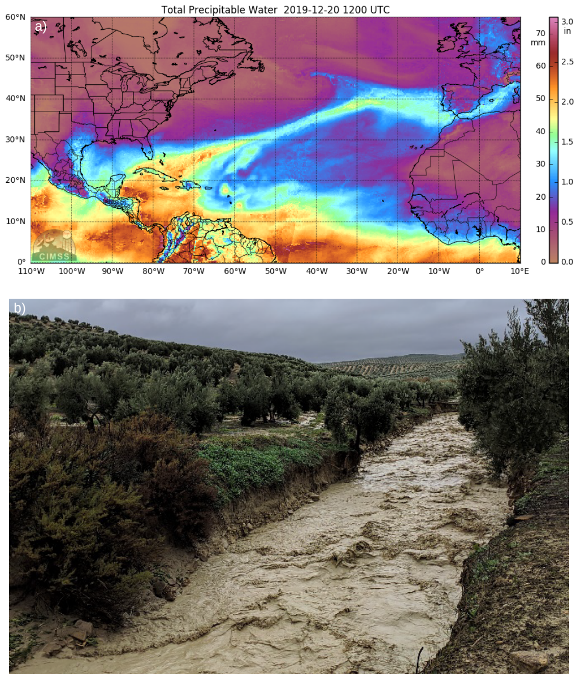
Figura 9. (a) Agua precipitable total (mm) a las 13 horas del día 20 de diciembre de 2019. Se aprecia un río atmosférico de alta humedad desde el mar Caribe hasta la Península Ibérica (Fuente: CIMSS). (b) Gran volumen de escorrentía transportado durante el mismo día en un pequeño cauce tributario ( A_{\text{drain}} < 10 \text{ km}^2 ) del Arroyo Salado de Porcuna.
