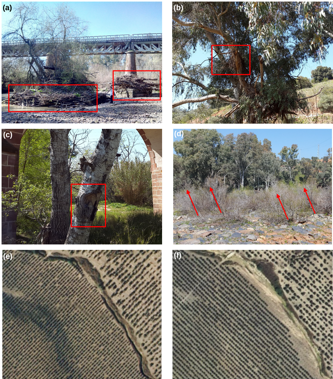
Figura 19. Acumulación de elementos ligeros transportados por el flujo de agua durante la inundación (a – b) sobre vegetación de ribera del río Guadalquivir. (c) Muesca de un ejemplar arbóreo causada por el impacto con un material pesado transportado. (d) Imbricación botánica en el sentido del flujo de inundación de unos ejemplares de Tamarix sp. Cultivo de Olea Europaea en un momento previo (e) y posterior (f) a la inundación relámpago de 2009 en el arroyo de Ibros. Nótese la importante eliminación de ejemplares próximos al cauce.
