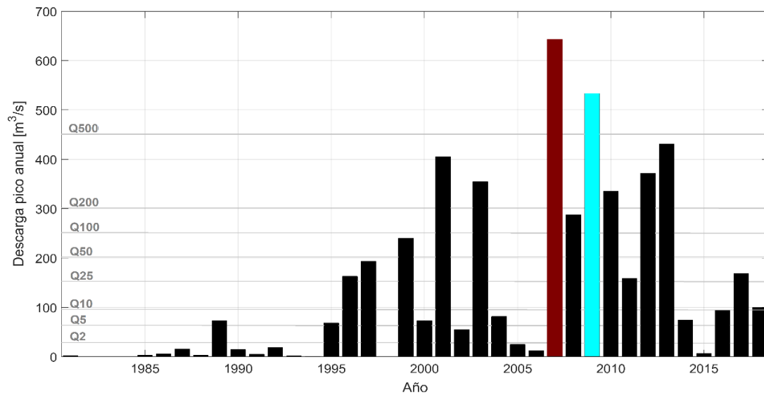
Figura 13. Descargas máximas anuales en el período 1981 – 2019 en la cuenca del Arroyo Salado de Porcuna (estación de aforo 5142). En color marrón y azul se destacan los eventos de mayor magnitud y el seleccionado para el estudio, respectivamente. Las líneas horizontales grises indican el caudal en diferentes períodos de retorno, dado por CAUMAX (Álvarez et al., 2012) para la misma sección (Moral-Erencia et al., 2020).
