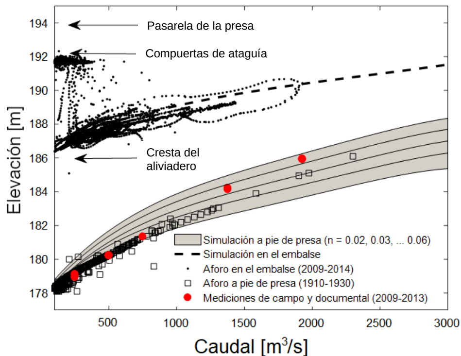
Figura 30. Curva caudal-cota de agua para los sectores situados aguas arriba y abajo de la presa de Marmolejo (Bohorquez & del Moral-Erencia, 2017).
