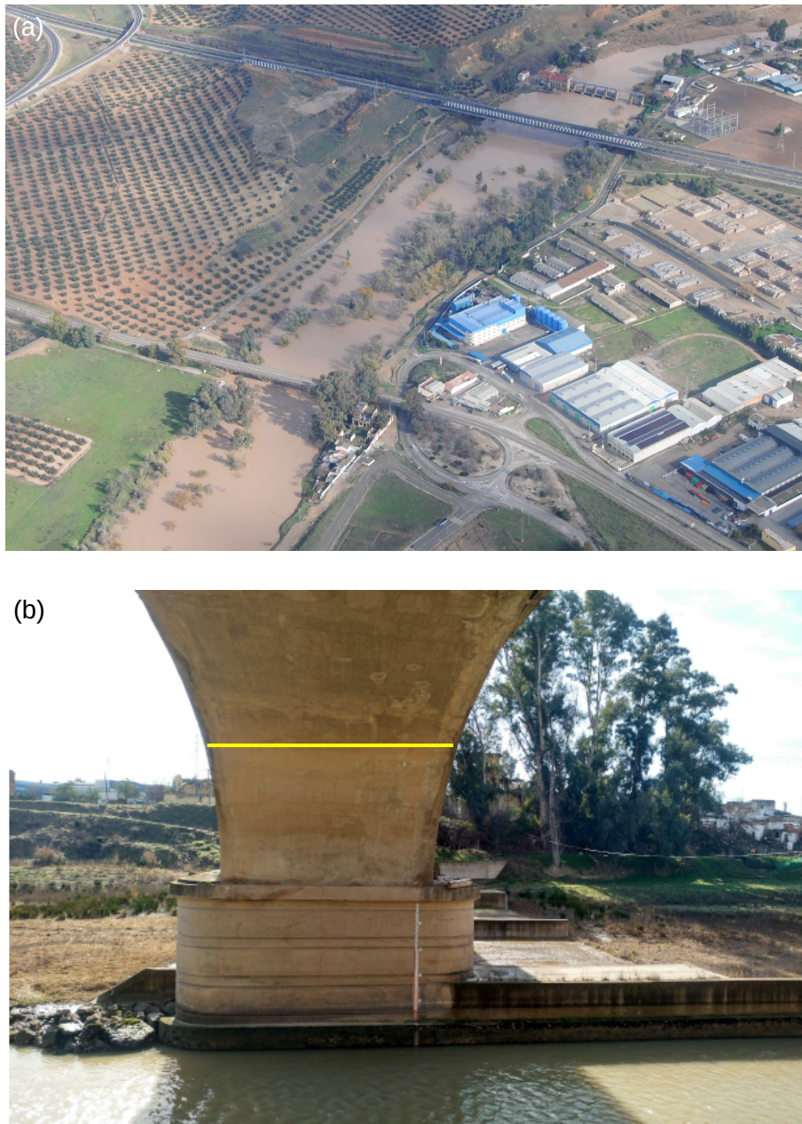
Figura 26. (a) Imagen de helicóptero de la entrada del tramo Mengíbar-Espelúy, empleada para la delimitación del nivel de agua de la inundación. (b) Marcas de sedimento fino sobre un puente anexo a la localidad de Mengíbar (Jaén) que permiten obtener un nivel máximo de la inundación.
