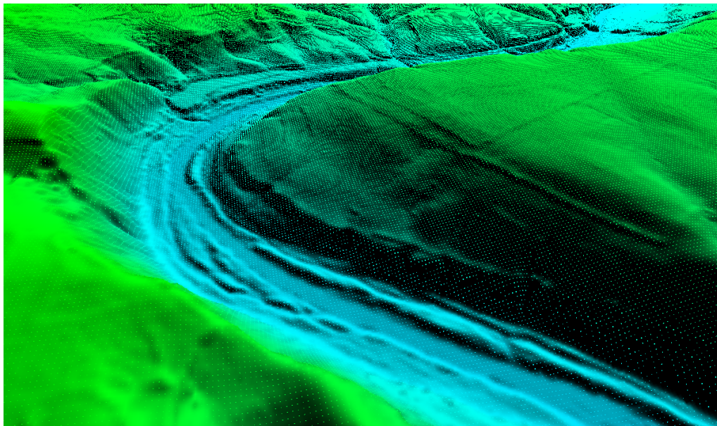
Figura 20. Modelo digital del terreno de gran detalle construido en el valle confinado de salida del sector Mengíbar-Marmolejo a partir de una nube de puntos LiDAR (superpuesta).
