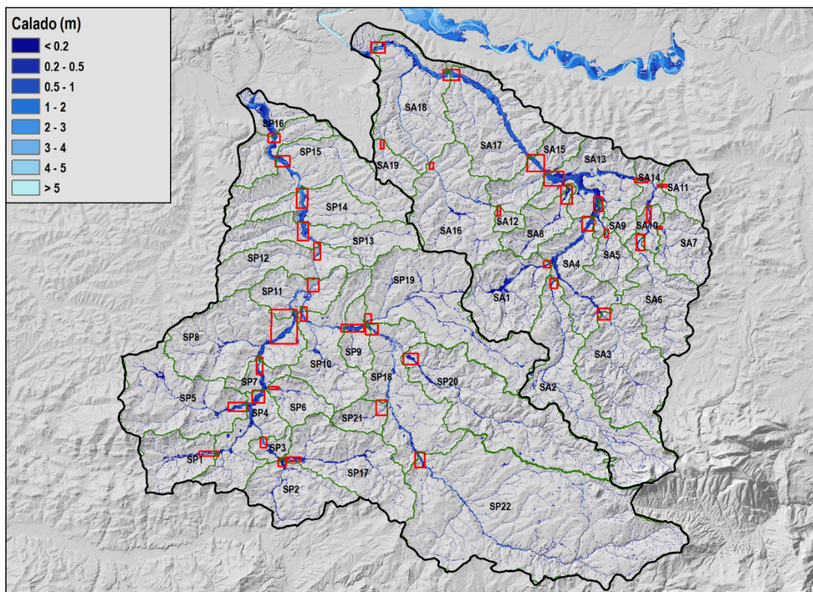
Figura 35. Calado simulado tras la aplicación del método directo mediante el modelo hidrológico distribuido, usando una precipitación de PMP_a de 2,9 mm·h -1 en SP y 5,4 mm·h -1 en SA. Los perímetros en color verde designan la división de subcuencas utilizadas para la verificación del cálculo hidrológico y la realización del cálculo refinado (Moral-Erencia et al., 2021, enviado).
