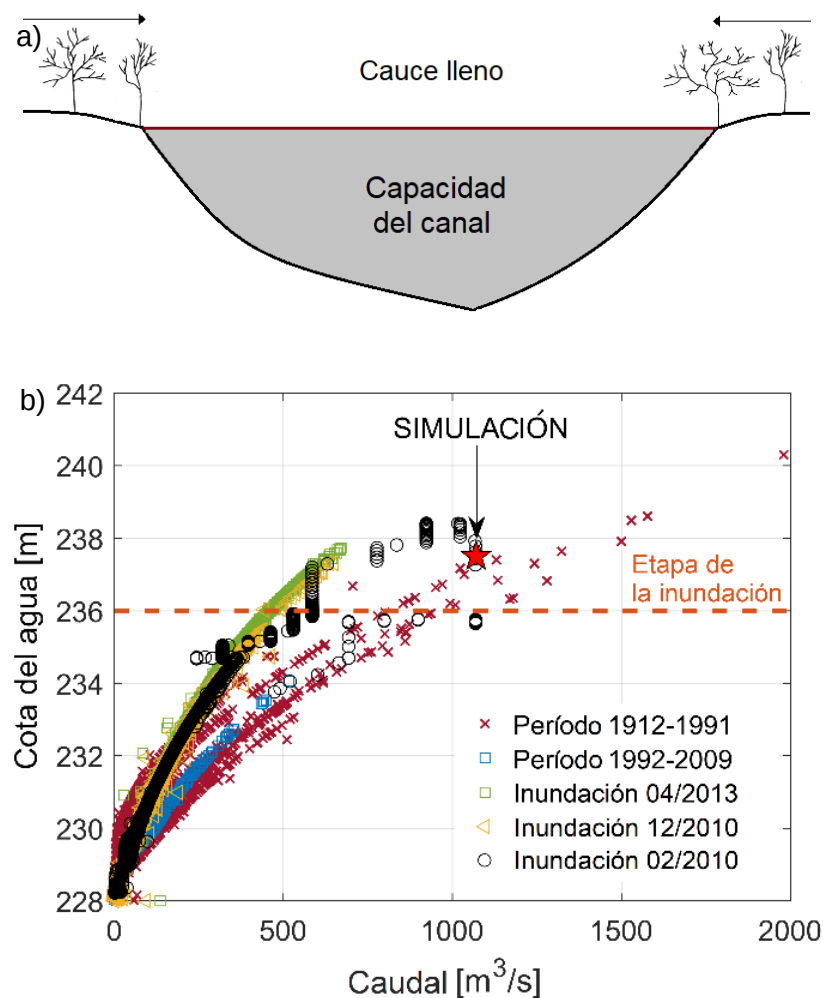
Figura 28. (a) Diagrama esquemático de la definición de capacidad de canal de un curso fluvial. Las flechas indican el proceso de colonización de la vegetación no flexible observado que conlleva su reducción en el río Guadalquivir. (b) Curva de gasto de la estación de aforo de Mengíbar en el período 1912 – 2013. Nótese la sobreelevación de los eventos modernos respecto al período 1912 – 1991. ★ indica la cota de agua de la simulación numérica bidimensional para Q = 1.070 \text{ m}^3 \cdot \text{s}^{-1} (caudal pico de la inundación de febrero de 2010) (Bohorquez & del Moral-Erencia, 2017).
