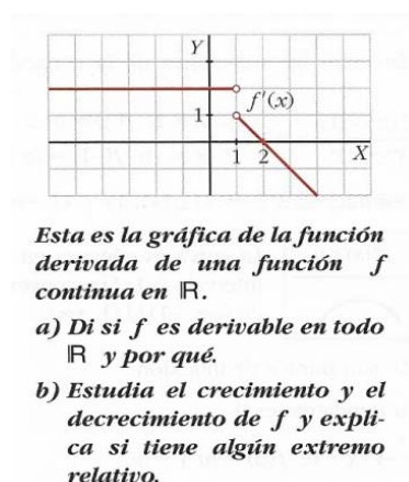
Figura 4.3: Relación del extremo relativo en la gráfica de la función derivada
