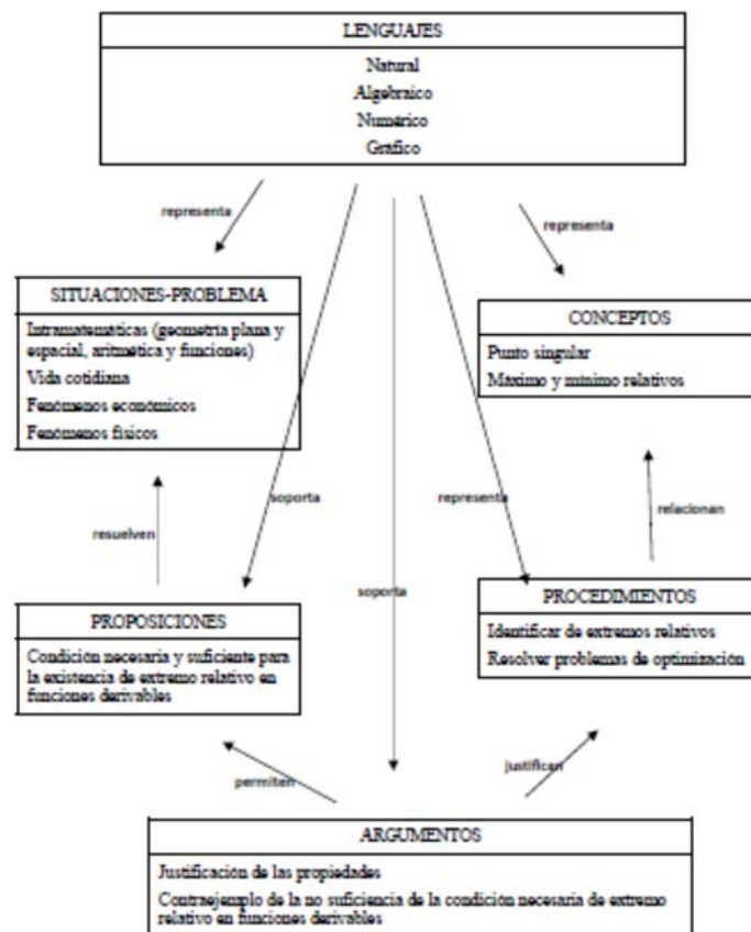
Figura 4.15: Configuración epistémica de la optimización del libro de texto T1
