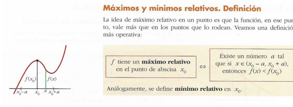
Figura 4.8: Definición de extremo relativo según CE-O utilizando tres RRS
