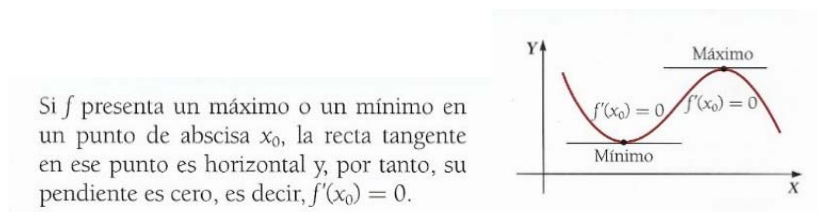
Figura 4.25: Extremo relativo según CE-T
