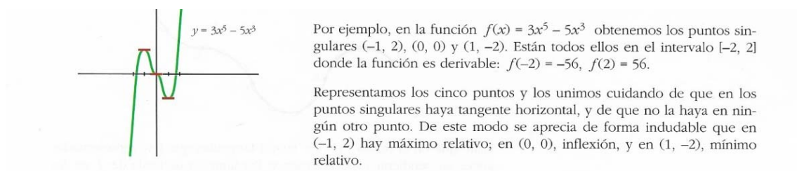
Figura 4.11: Ejemplo donde se identifican los extremos relativos según CE-T
