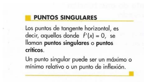
Figura 4.7: Definición punto singular o punto crítico
