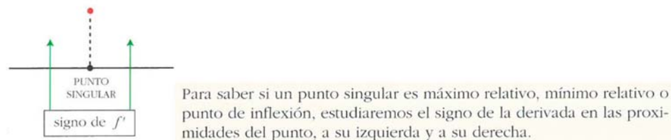
Figura 4.6: Procedimiento para clasificar un punto singular según CE-1D
