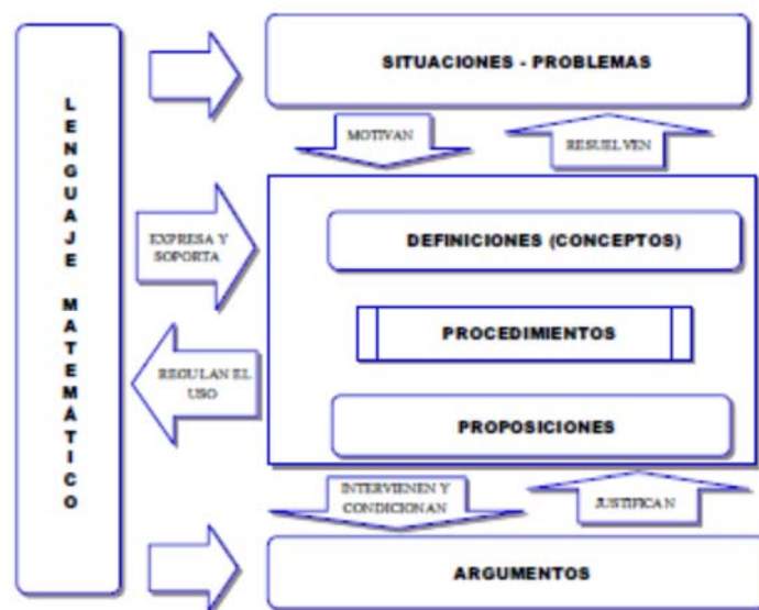
Figura 2.2: Configuración de las entidades primarias matemáticas
