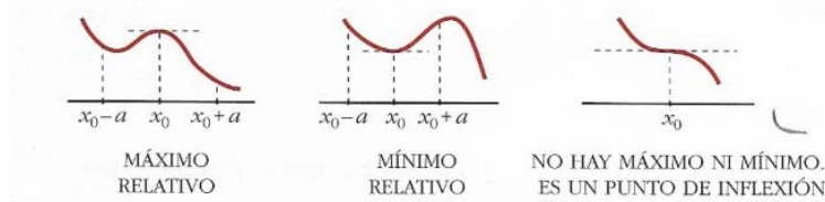
Figura 4.13: Clasificación puntos críticos según CE-T
