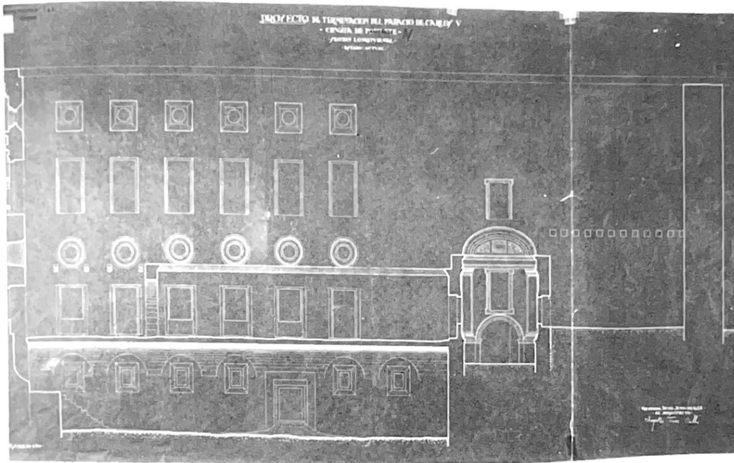
3. Plano de L. Torres Balbás del corte longitudinal de la crujía norte del Palacio de Carlos V. Foto: Valentín García Baca
