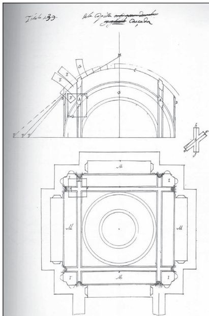
“Capilla Cruzada” (Alonso d Vandelvira, “Libro de Cortes de Piedra”
