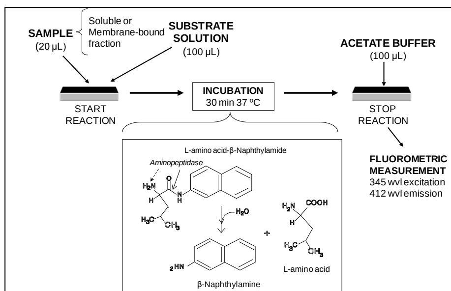
Figura 3. Esquema que indica el procedimiento seguido para la obtención de las fracciones soluble y unida a membrana, donde se determinaron, mediante fluorimetría, las diversas actividades enzimáticas y, mediante espectrofotometría, el contenido de proteínas (tomado de Ramírez y cols, 2011).
